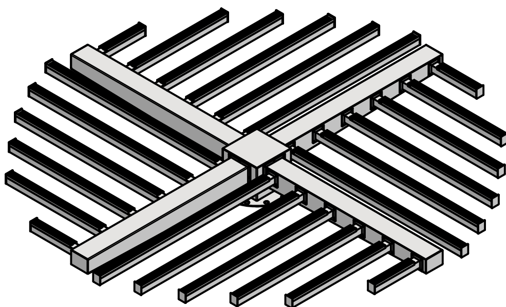
KND-2600 ДРС \Phi 2600 — общий вид 4 главных луча \times 6 ответвлений Масштаб видов 1:20, 1:18
